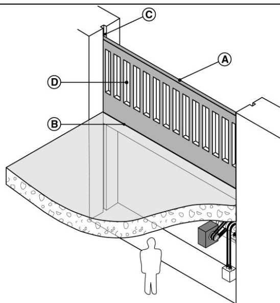
Gefahrstellen an kraftbetätigten Schiebetoren mit vertikaler Bewegung von unten nach oben (Abbildung 1).
